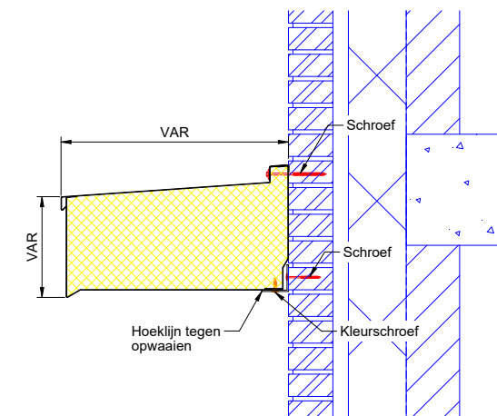
Detail gevelband
