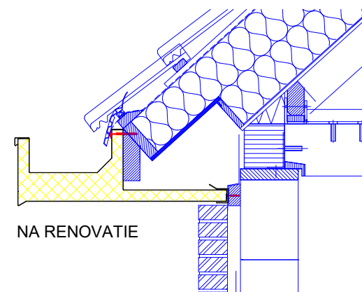
Detail renovatie
