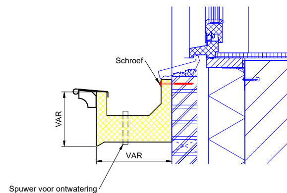
Detail bloembak
