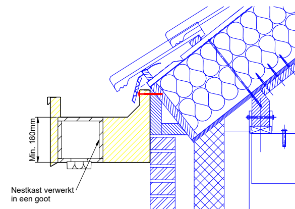
Detail nestkast
